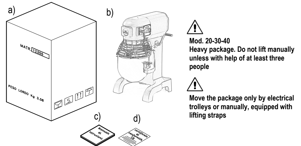
FIG. n.3 - Packaging description
